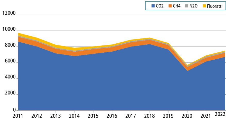
Gràfic I-11.1. Emissions dels GEH a les Balears (kt de CO2 equivalent) (2011-2022)
