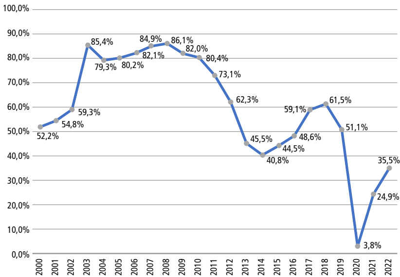
Gràfic I-11.2. Evolució de les emissions de gasos amb efecte d'hivernacle respecte del 1990 (%)
